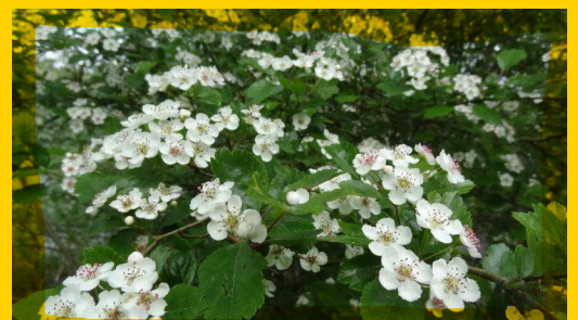
Crataegus monogyna
