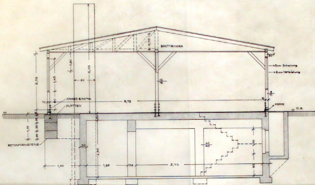
Schnitt M. 1:50
