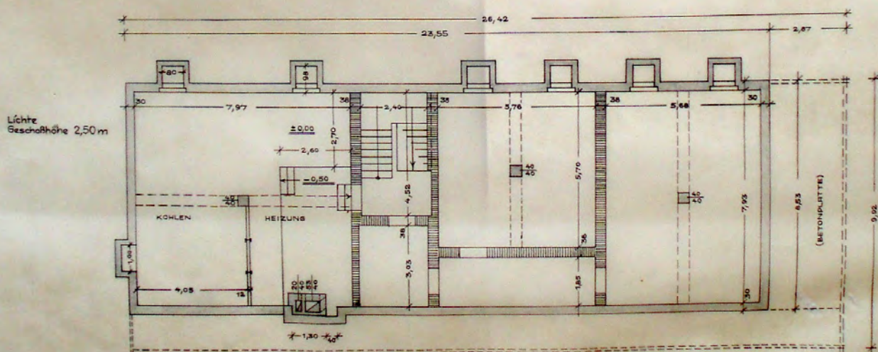
Grundriß Kellergeschoß M. 1:100
